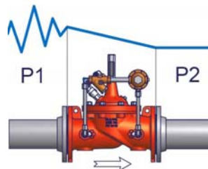
Regelverhalten
